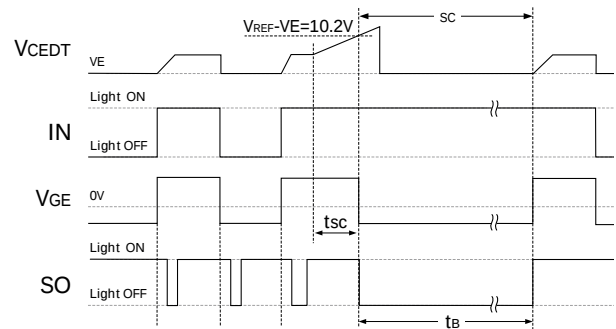
图 6. 保护信号输出逻辑
