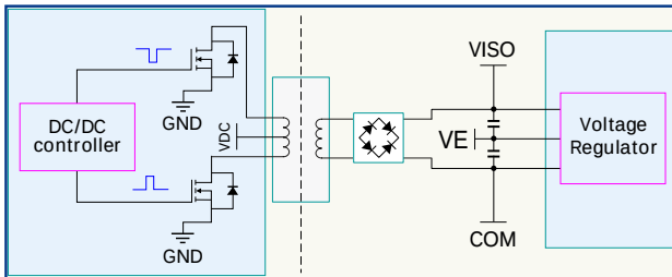
图 3. 供电电路
