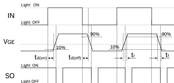
图 5. 输入 / 输出逻辑时序
