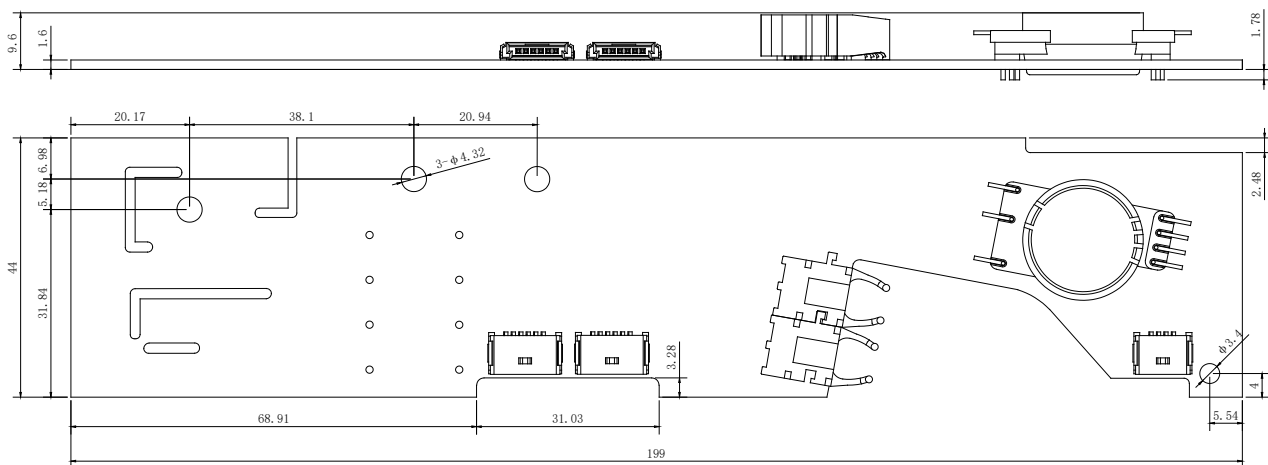
图 13. 1QP0635Vxx 机械结构图
