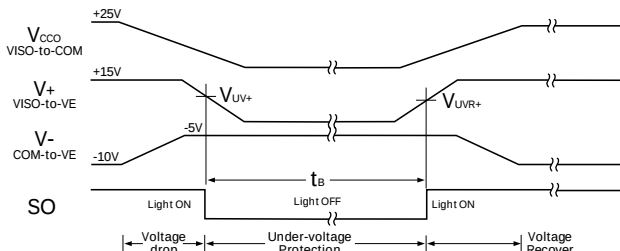
图 4. 副边欠压保护逻辑
