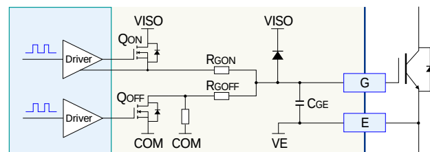
图 7. 门极驱动电路
