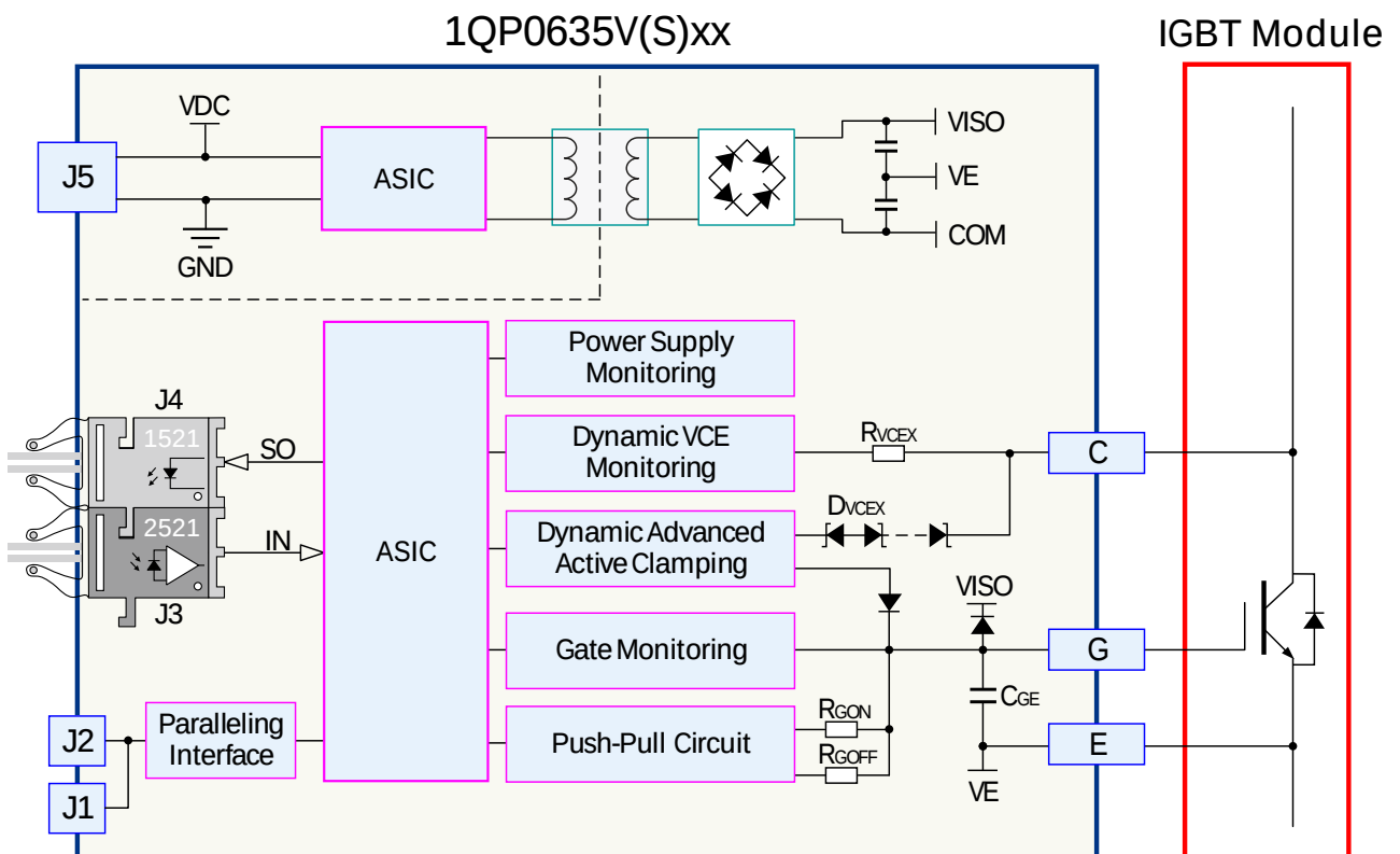
图 1. 1QP0635V(S)xx 原理框图
