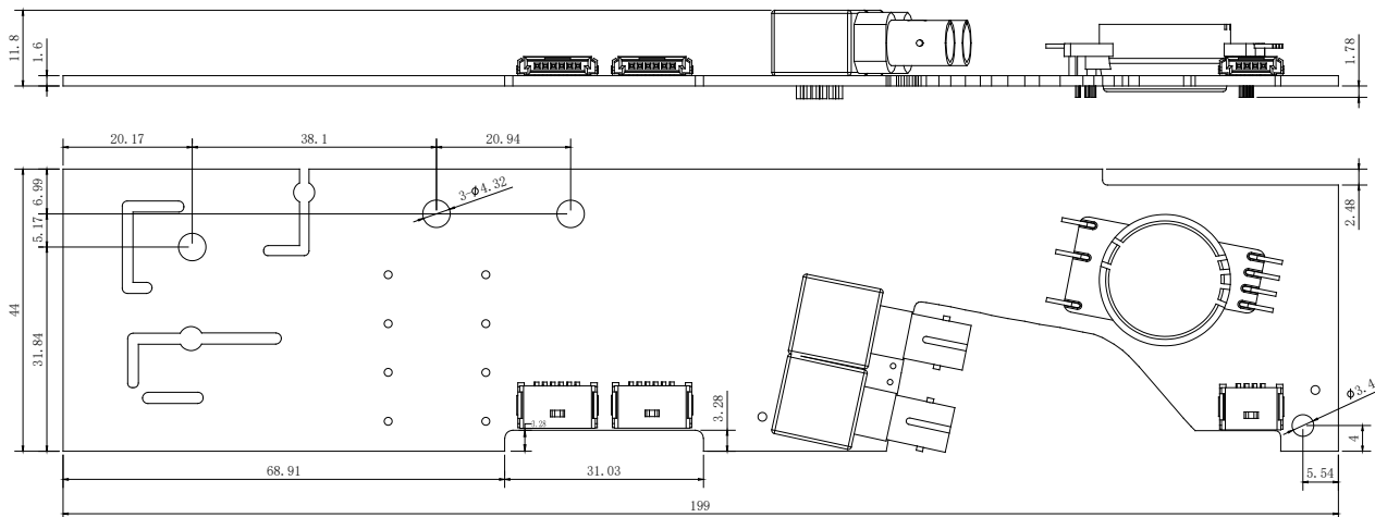
图 14. 1QP0635Sxx 机械结构图
