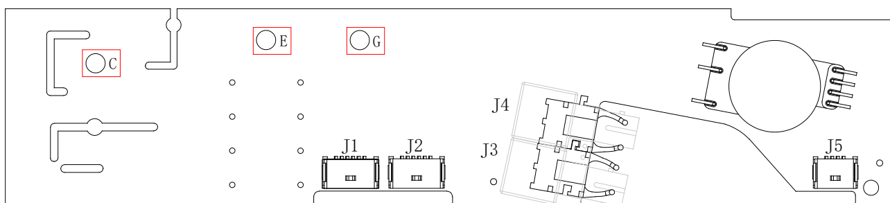
图 2. 1QP0635V(S)xx 插座位置
