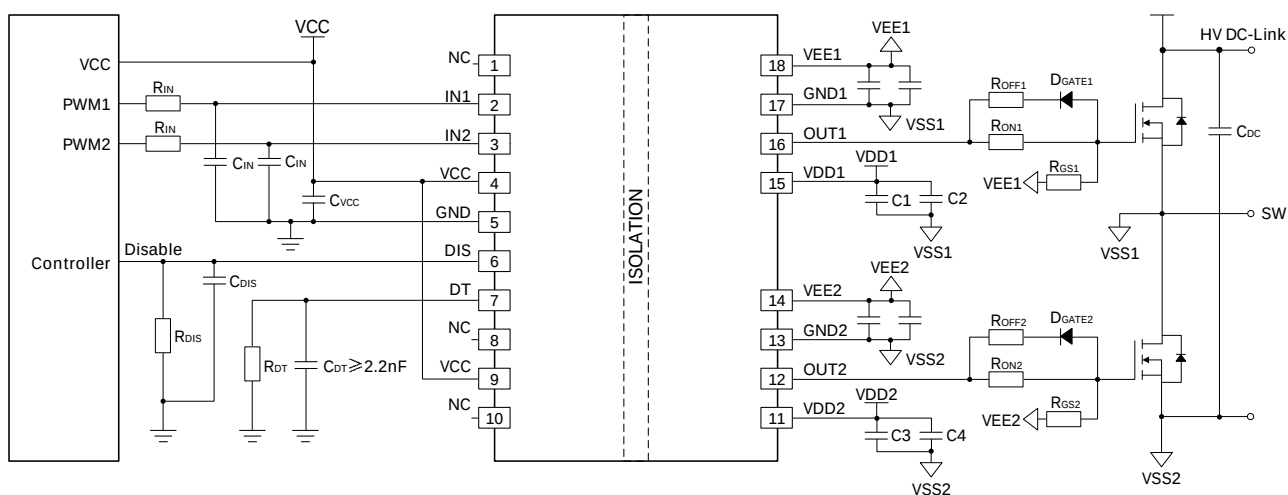
图 31 BTD25350MEx 典型应用
