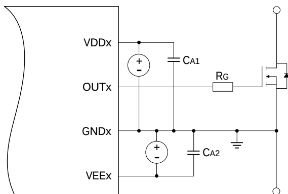
图 33 双电源方案
