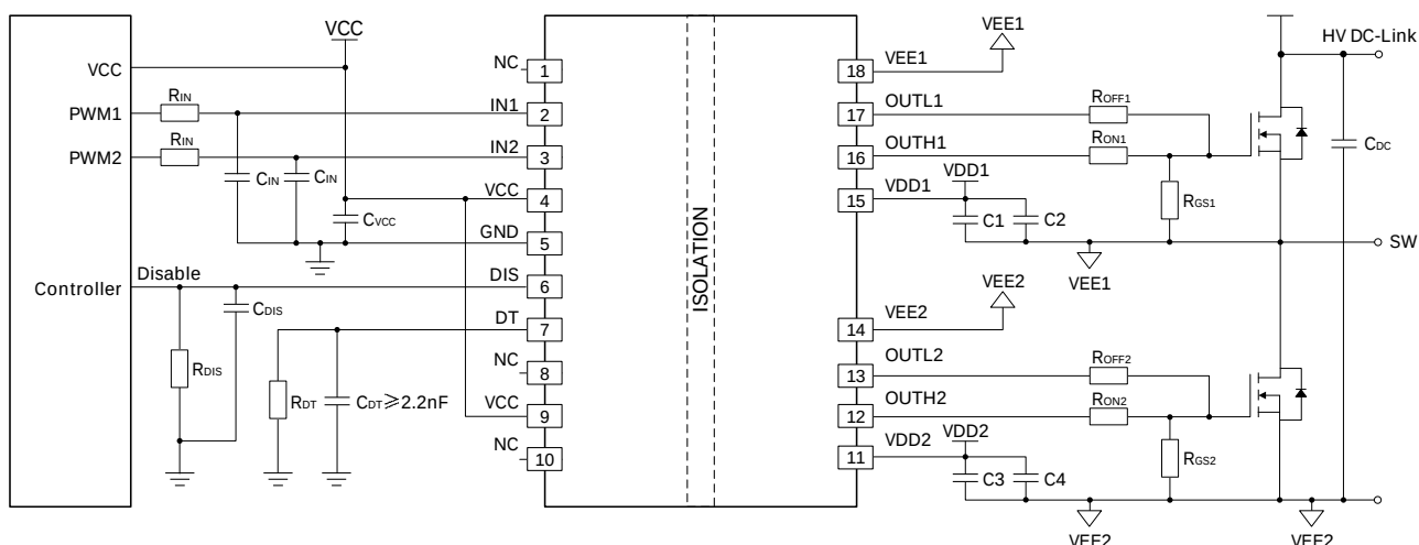
图 30 BTD25350MSx 典型应用
