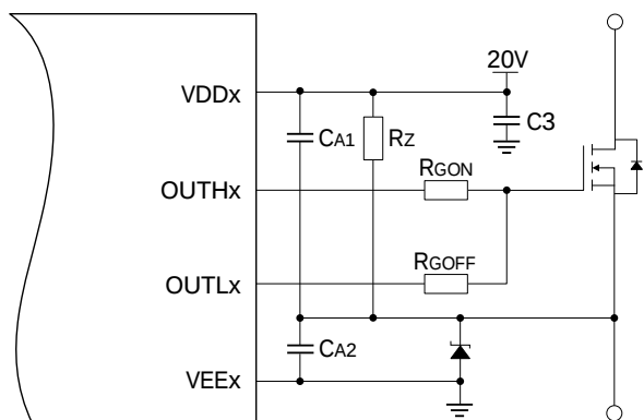
图 32 稳压管方案
