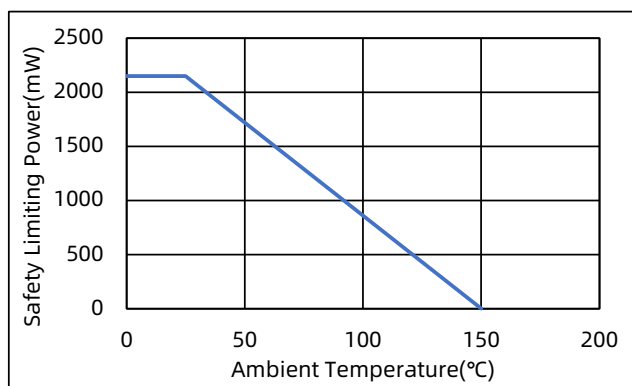
图 5 安全功率的温度降额曲线
