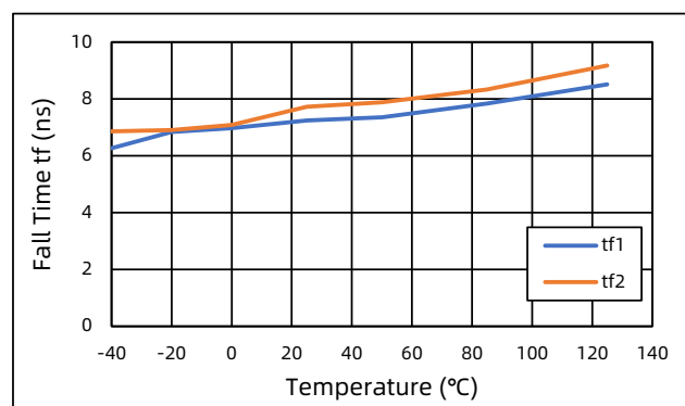
图 14 下降时间 vs. 温度 (1nF 负载)
