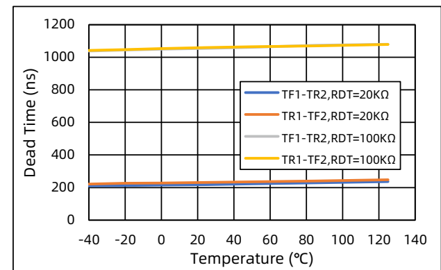
图 22 死区时间 vs. 温度 ( R_{DT}=20k\Omega/100k\Omega )
