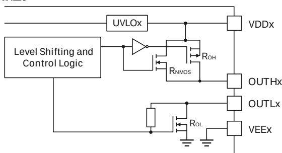
图 26 输出特性示意图
