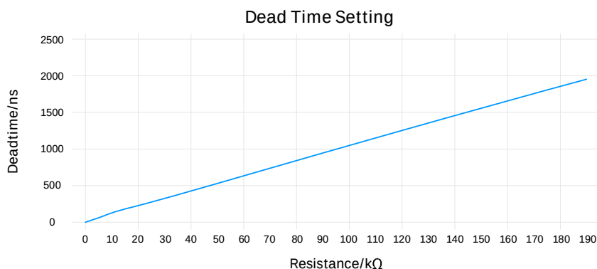
图 25 死区时间曲线图
