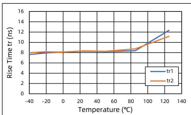
图 13 上升时间 vs. 温度 (1nF 负载)
