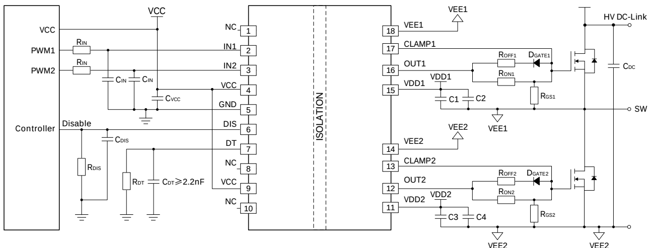
图 29 BTD25350MMx 典型应用
