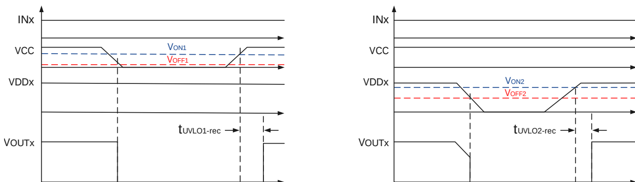
图 27 输出特性示意图
