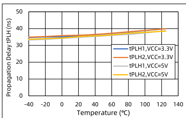
图 15 传输延时 vs. 温度 (1nF 负载)
