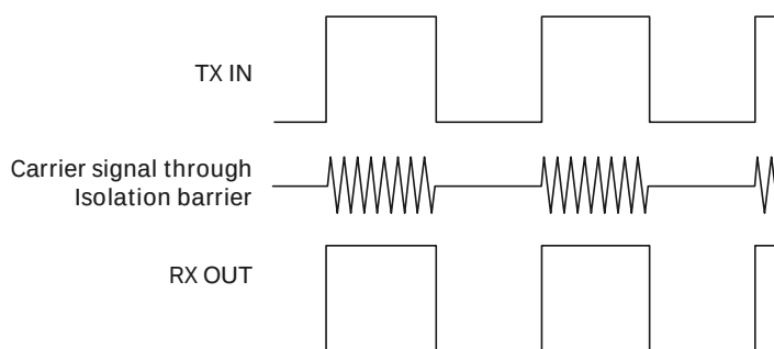
图 24 OOK 调制解调示意图
