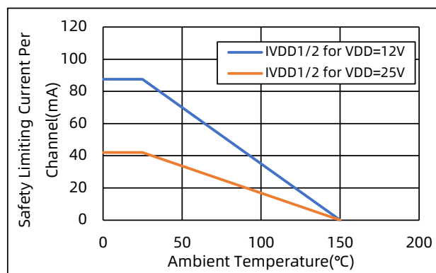
图 6 安全电流的温度降额曲线
