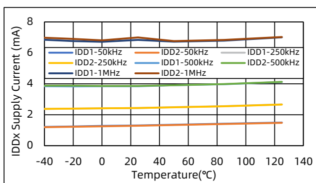
图 9 单通道电源电流 vs. 温度 (无负载, 不同的开关频率)
