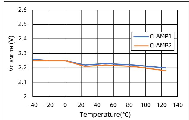
图 18 V_{CLAMP-TH} vs. 温度
