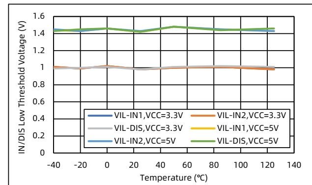
图 20 IN/DIS 低电平阈值 vs. 温度
