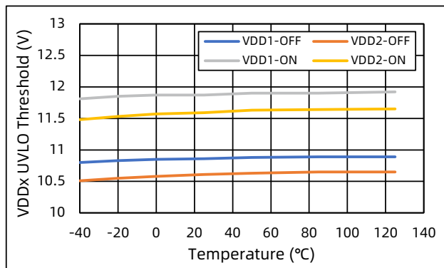
图 19 副边欠压阈值 vs. 温度
