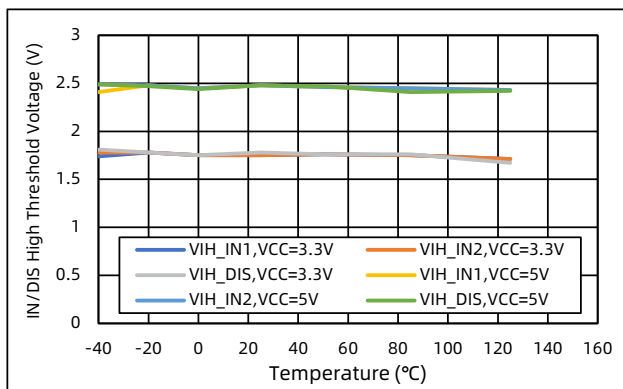
图 21 IN/DIS 高电平阈值 vs. 温度
