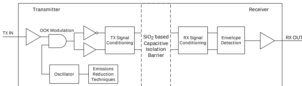
图 23 隔离传输示意图
