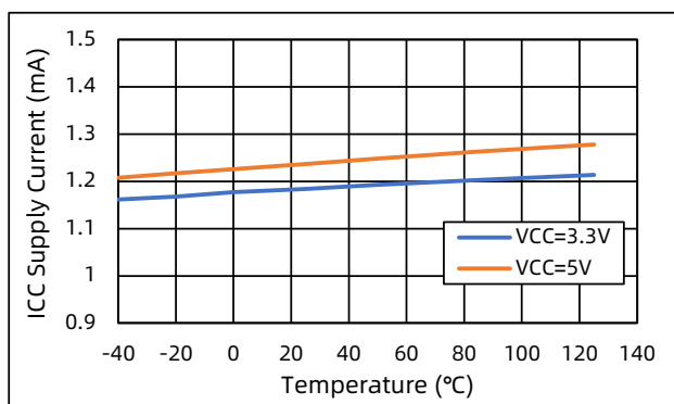
图 11 原边供电 I_{VCC} 静态电流 vs. 温度 (空载, 输入低电平)
