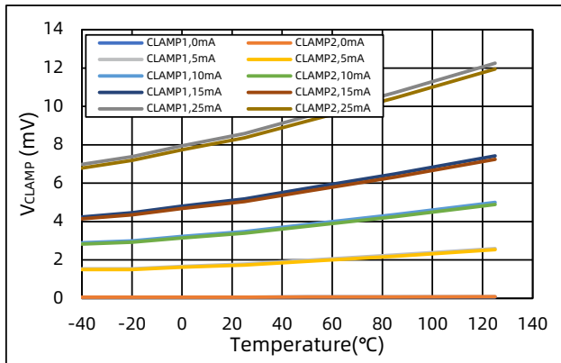
图 17 V_{CLAMP} vs. 温度 (输入低电平)
