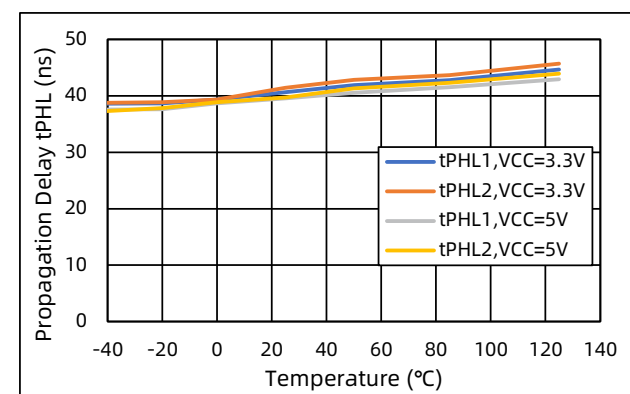
图 16 传输延时 vs. 温度 (1nF 负载)
