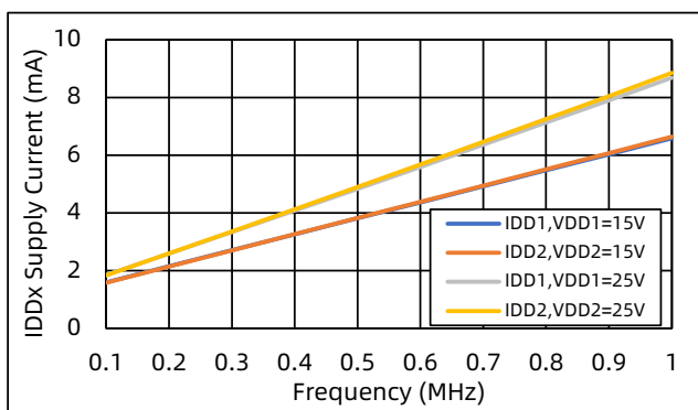
图 7 单通道电流消耗 vs. 频率 (空载, V_{DD} = 12\text{V} 或 25\text{V} )
