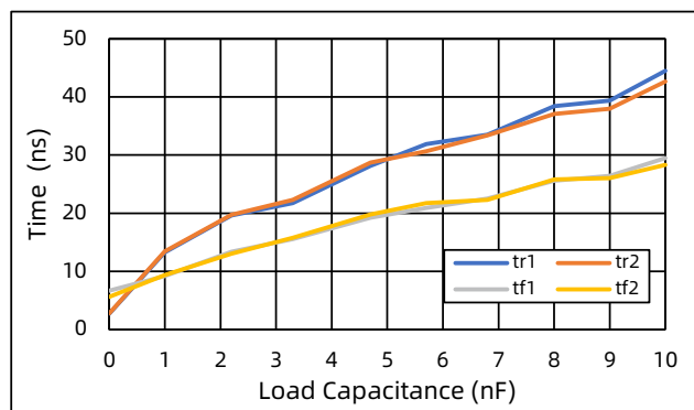
图 12 上升和下降时间 vs. 负载 ( V_{VDD1/2} = 15V )
