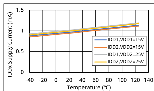
图 10 副边供电每通道静态电流 vs. 温度 (空载, 输入低电平)
