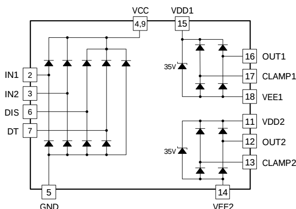
图 28 ESD 结构示意图
