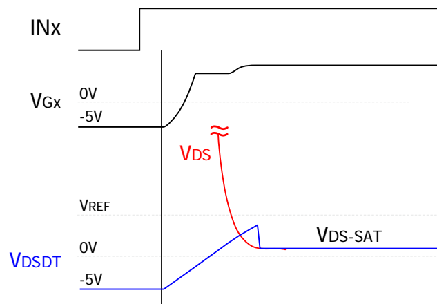
图 13. 正常开通时 V_{DS\text{DT}} 信号波形图
