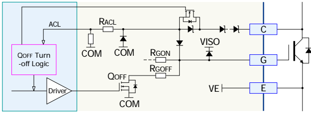
图 6 动态高级有源钳位电路图
