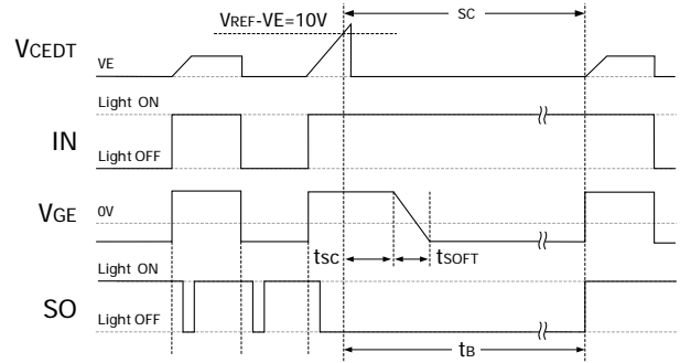
图 4 保护信号输出逻辑
