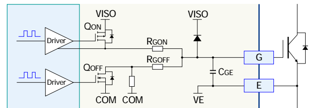
图 5 门极驱动电路图
