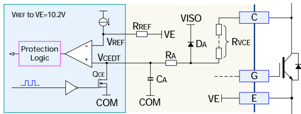
图 7 短路保护检测原理框图
