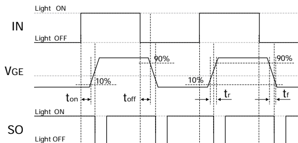
图 3 IN 输入逻辑
