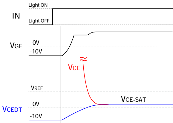
图 8 正常开通时 VCEDT 信号波形图
