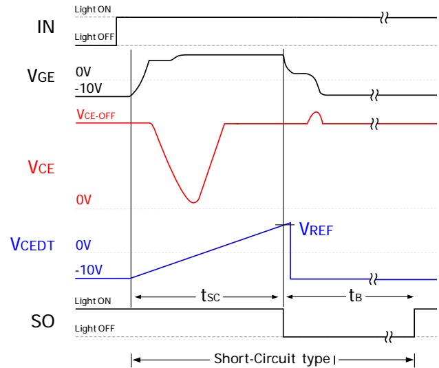
图 9 一类短路保护逻辑图
