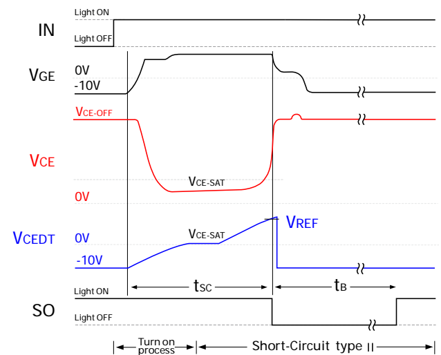
图 10 二类短路保护逻辑图
