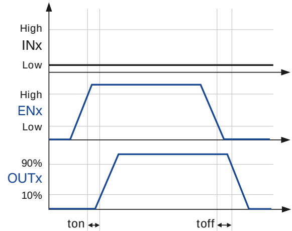
图 1-2 使能功能 (BTL27523)
