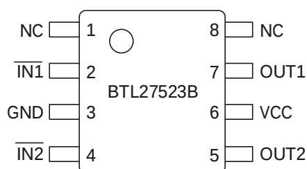
BTL27523B 管脚定义
