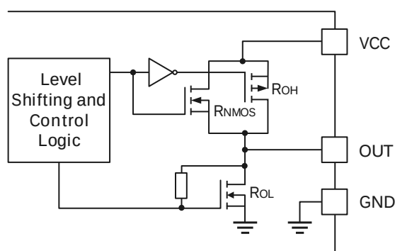
图 2 输出特性示意图
