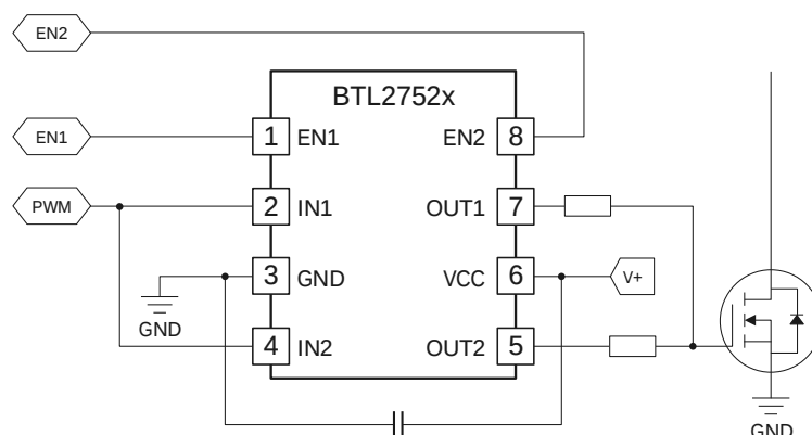
图 4-2 BTL2752x 通道并联应用图
