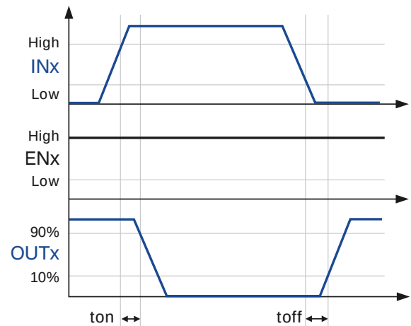
图 1-4 反相输入驱动器操作 (BTL27523)
