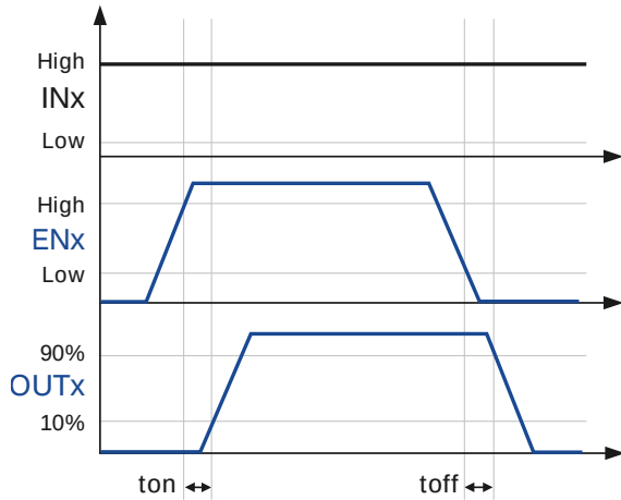
图 1-1 使能功能 (BTL27524)
