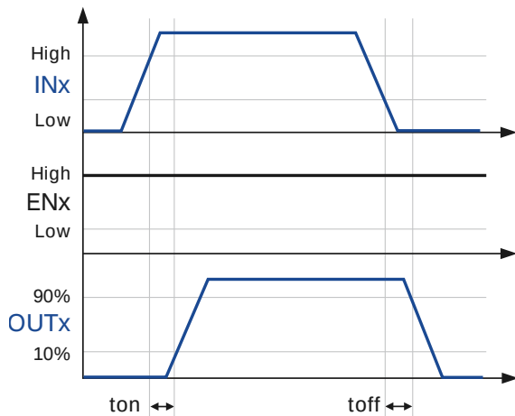
图 1-3 同相输入驱动器操作 (BTL27524)
