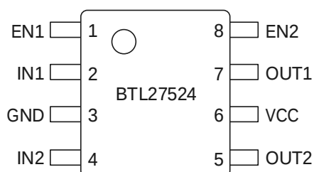
BTL27524 管脚定义
