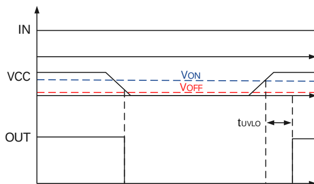
图 3 欠压保护示意图
