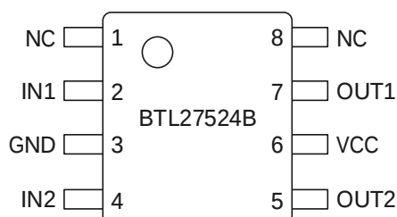
BTL27524B 管脚定义
