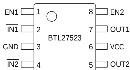
BTL27523 管脚定义
