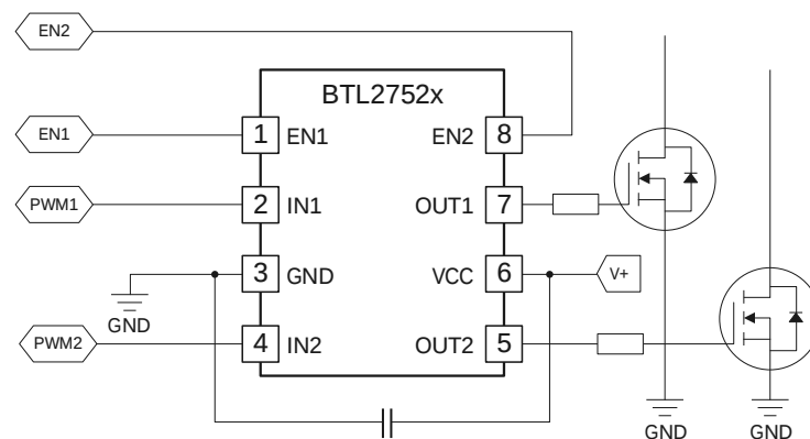
图 4-1 BTL2752x 典型应用图
