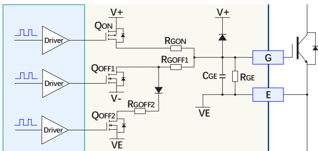
图 8 米勒钳位电路原理框图
