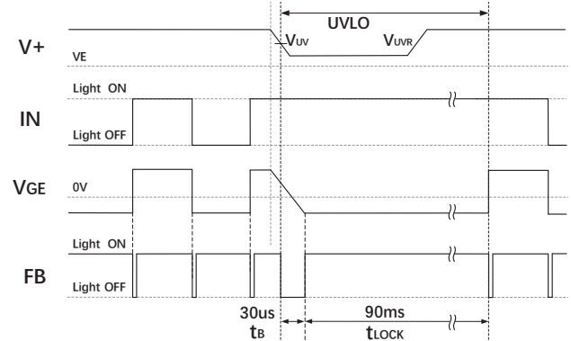
图 4 保护信号输出逻辑
