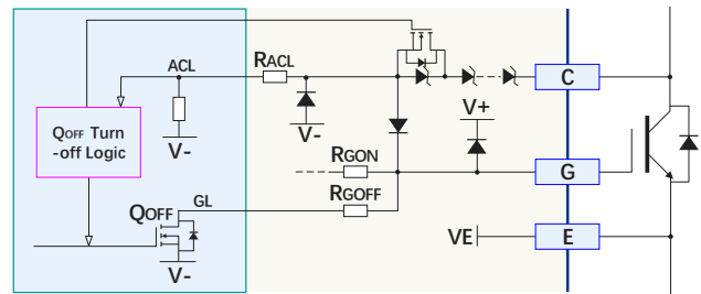
图 9 动态有源钳位电路原理框图
