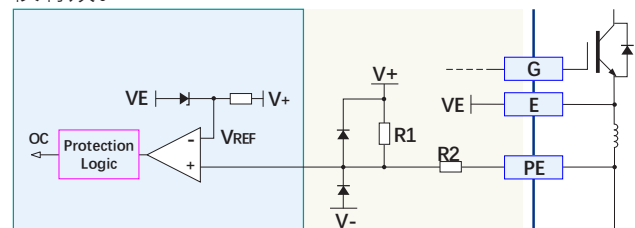
图 10 di/dt 短路保护检测原理框图
