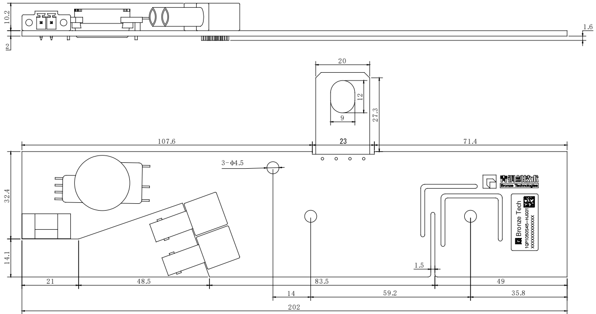
1QP1050S45-HJG01 机械尺寸图
