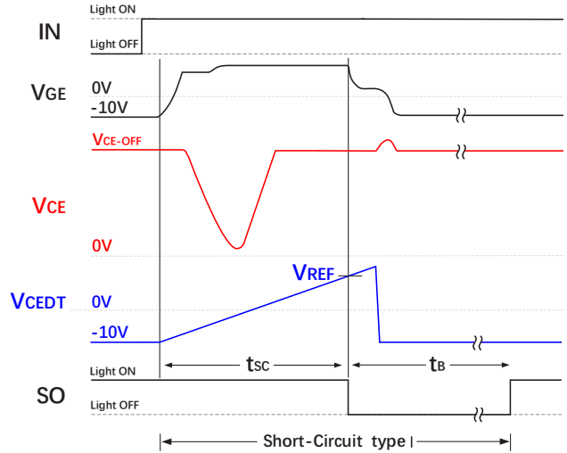
图 13 一类短路保护逻辑图
