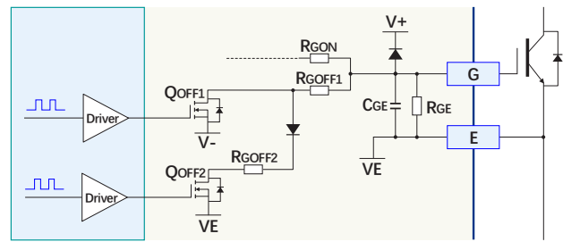
图 15 软关断示意图
