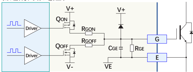
图 7 门极驱动电路
