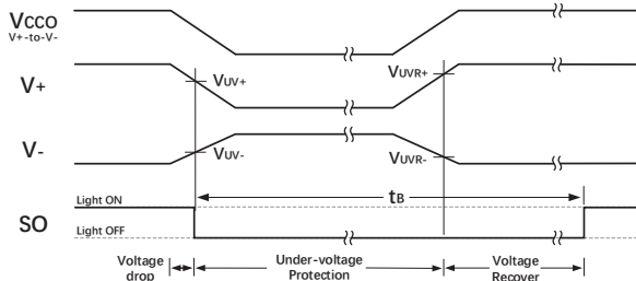
图 2 副边欠压保护逻辑图
