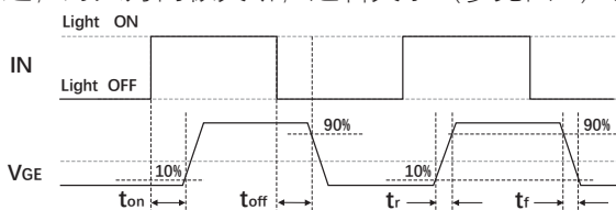
图 3 INx 输入逻辑图
