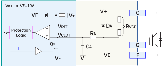
图 11 退饱和和短路保护检测原理框图
