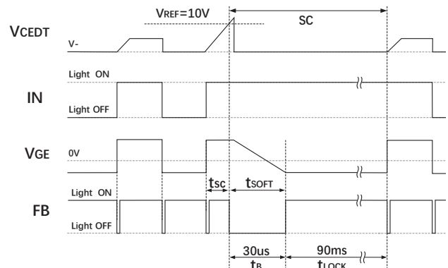
图 5 退饱和检测
