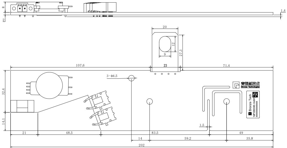
1QP1050V45-HJG01 机械尺寸图
