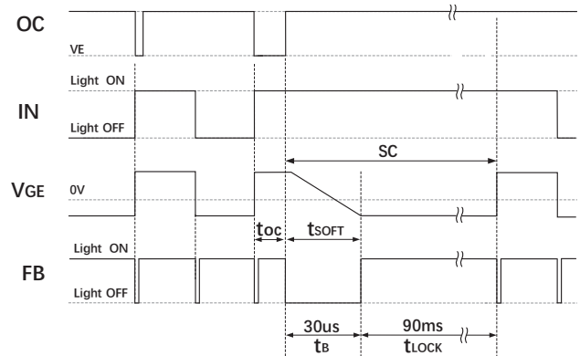
图 6 di/dt 检测
