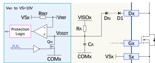
图 14 短路保护检测原理框图
