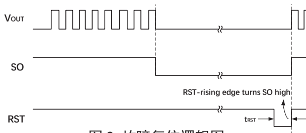
图 9 故障复位逻辑图
