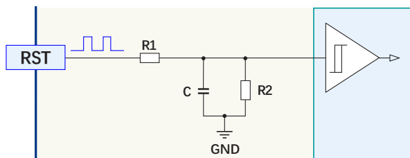
图 8 RST 输入电路图
