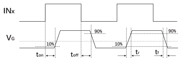
图 7 输入输出逻辑图
