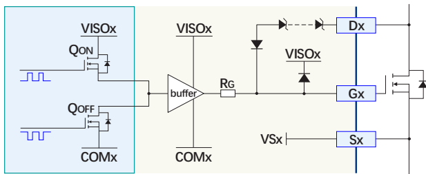
图 12 有源钳位电路原理框图
