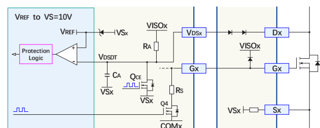
图 18 软关断原理框图
