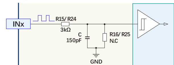
图 6 5/15V 输入电路图
