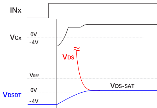
图 15 正常开通时 V_{DSDT} 信号波形图
