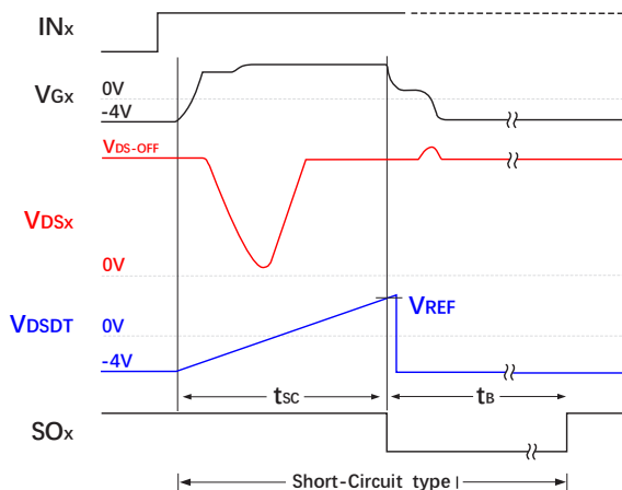
图 16 一类短路保护逻辑图
