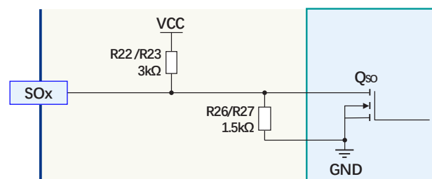
图 10 保护信号输出框图
