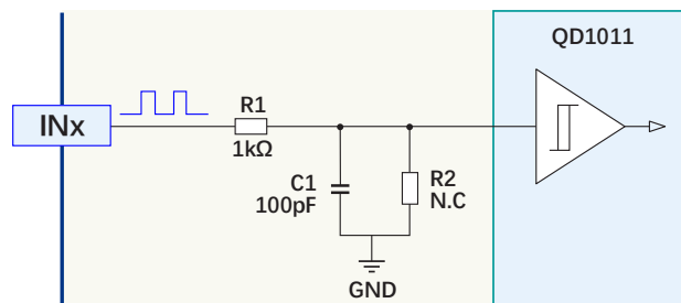
图 8 INx 输入电路图
