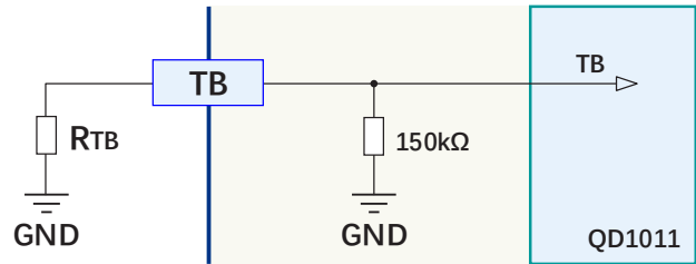
图 11 TB 管脚连接图
