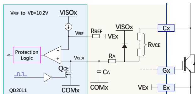
图 15 短路保护检测原理框图
