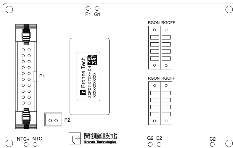
2QP0115Txx-CN 接口示意图
